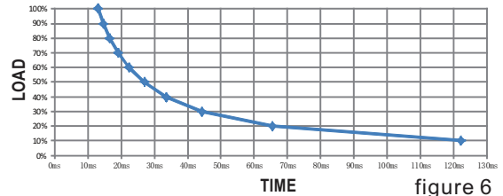
DDR-480D-24
