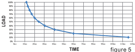
DDR-480D-12
